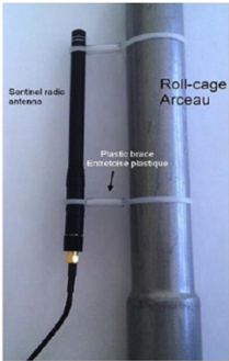
Рис. 6. Установка антенны
