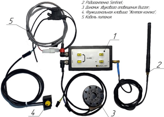
Рис. 5. Комплект системы Sentinel в сборе
